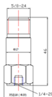
Dimensions
